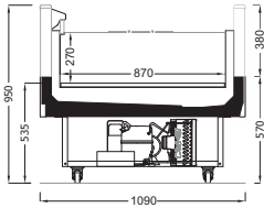
OCTOPUS V2 110 SLD
