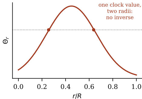
(d) non-monotone arrest: the equivalence fails
