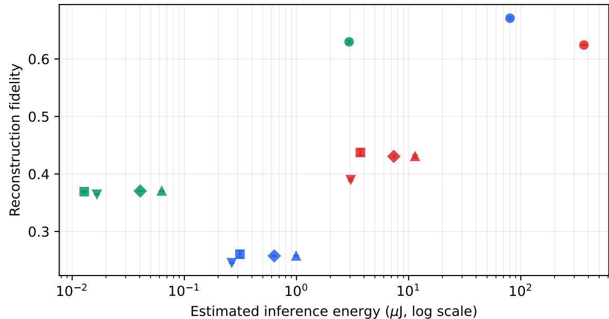
Haar Pure
