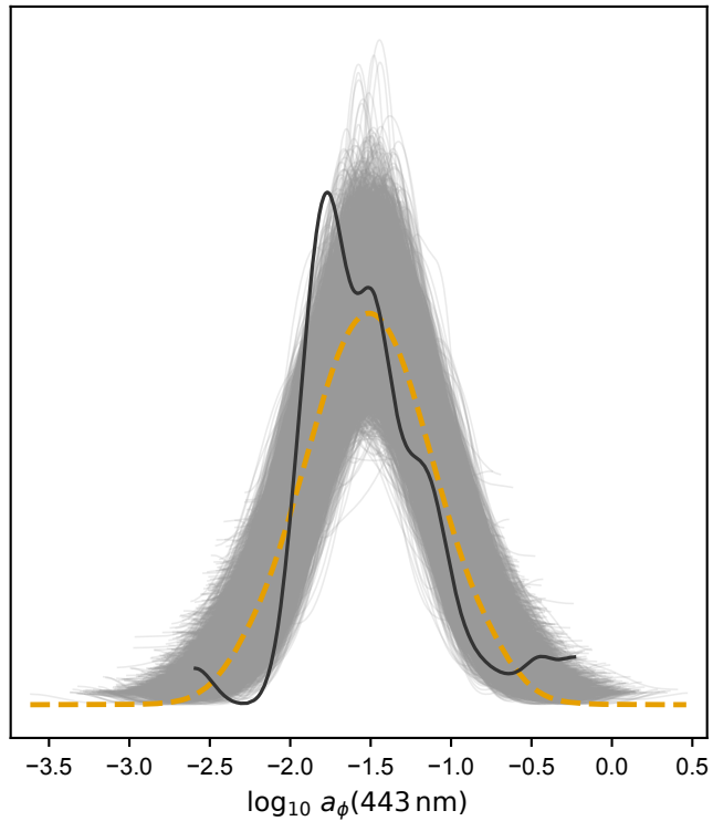
Posterior predictive
