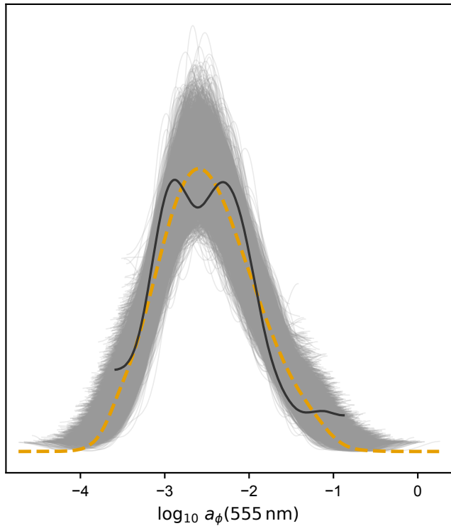
Posterior predictive
