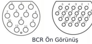
BCR Ön Görünüş
