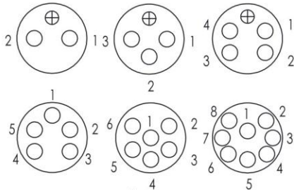
Erkek Ön Görünüş
