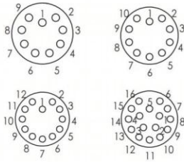
Erkek Ön Görünüş
