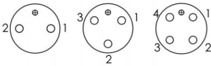
Erkek Ön Görünüş
