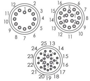
Erkek Ön Görünüş
