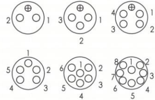
Erkek Ön Görünüş
