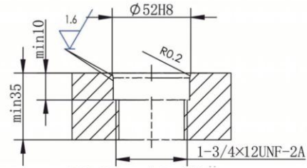
BCR Montaj Deliği
