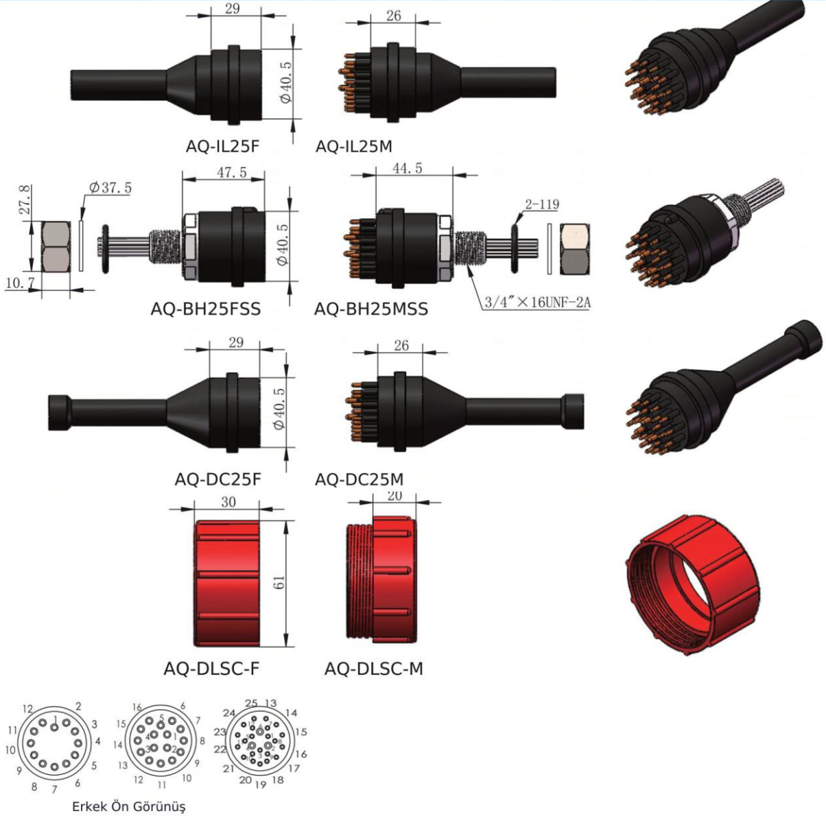
Erkek Ön Görünüş
