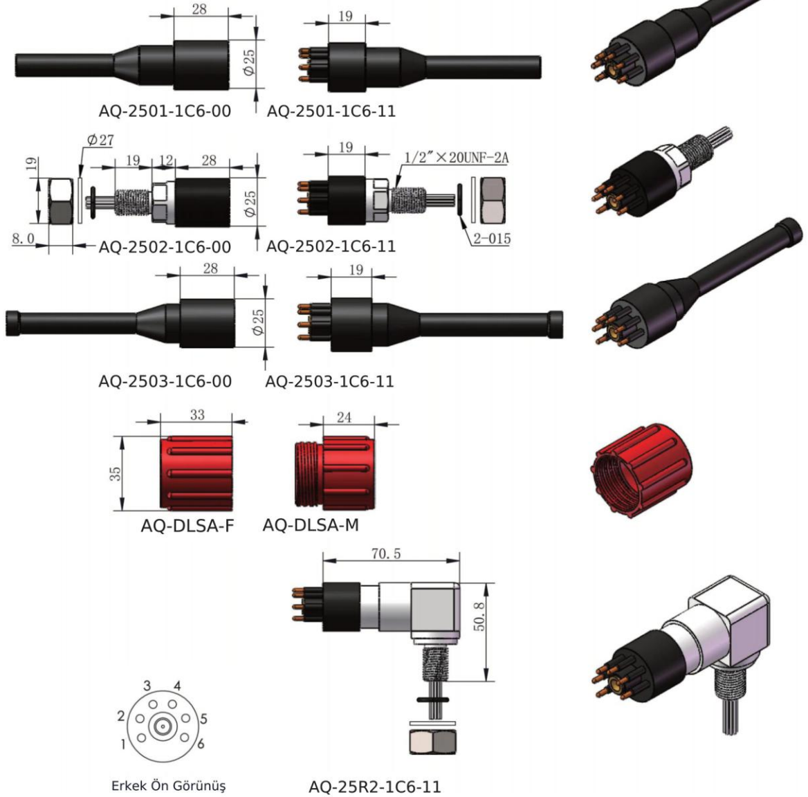
Erkek Ön Görünüş
