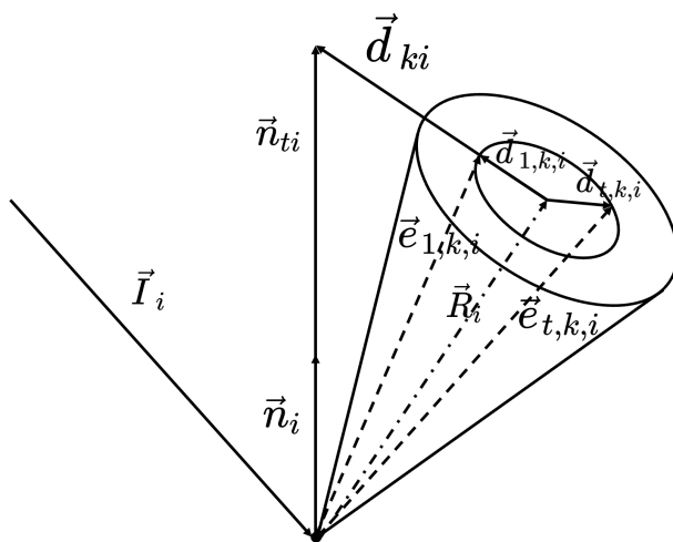
图 22: 离散光线向量 \vec{e}_{t,k,i} 计算示意图
