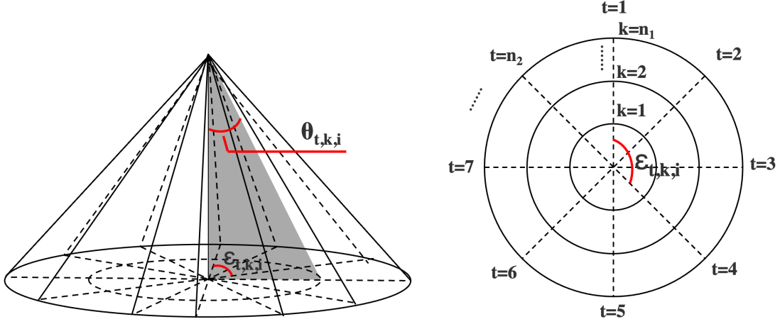
图 7: 锥形光线离散化示意图
