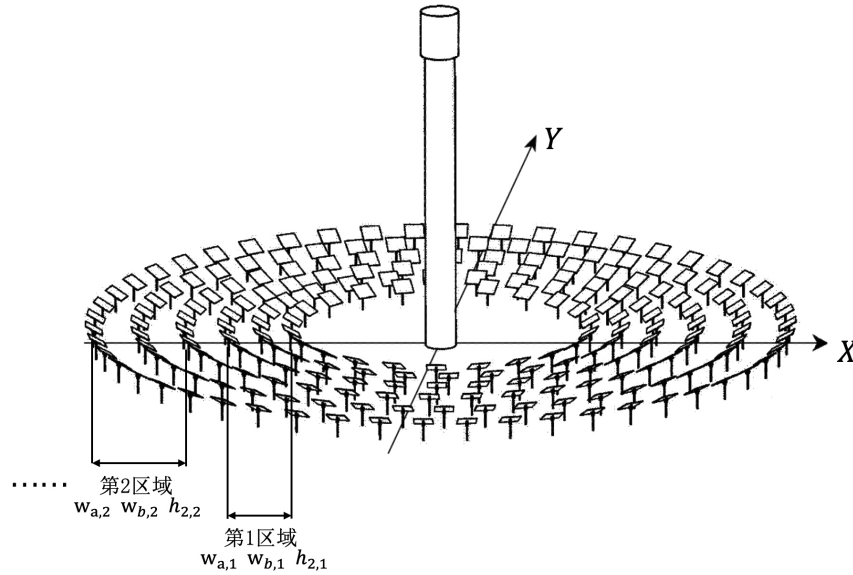
图 17: “定日镜规格分区域规划策略”示意图 [8]
