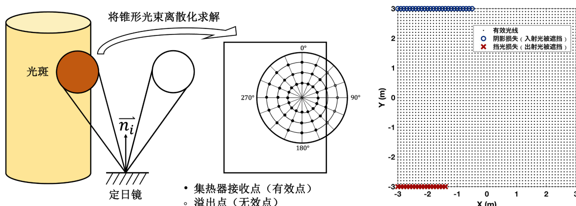
图 8: 集热器截断效率求解图 (左图) 与阴影遮挡效率求解图 (右图)
