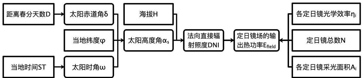
图 3: 影响 E_{field} 计算结果的变量逻辑框图
