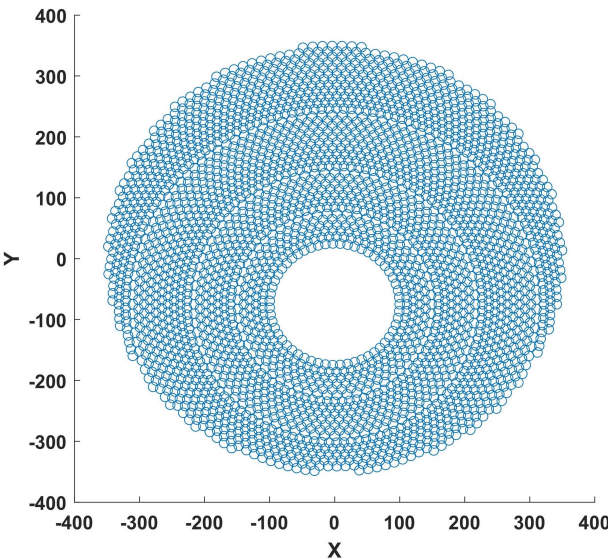
图 14: 吸收塔及定日镜布局可视化
