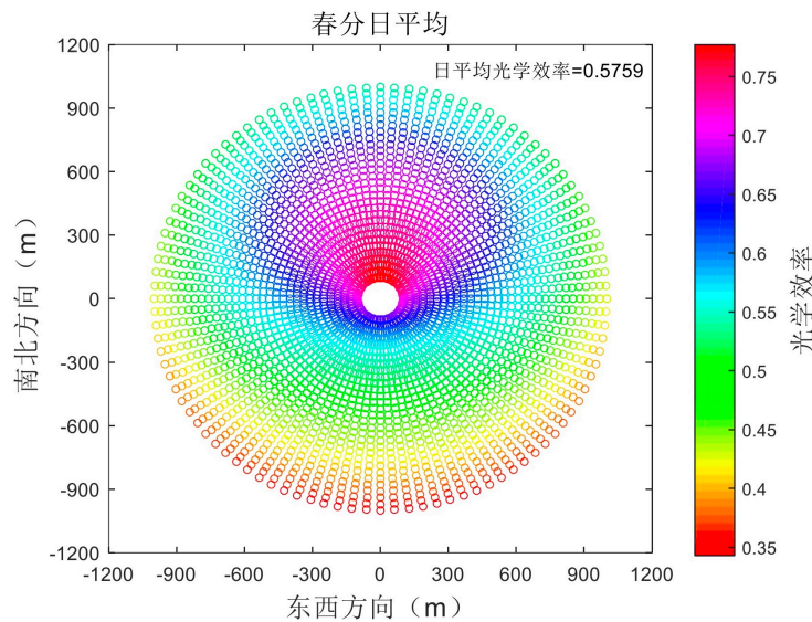
图 10: 春分日平均光学效率分布云图
