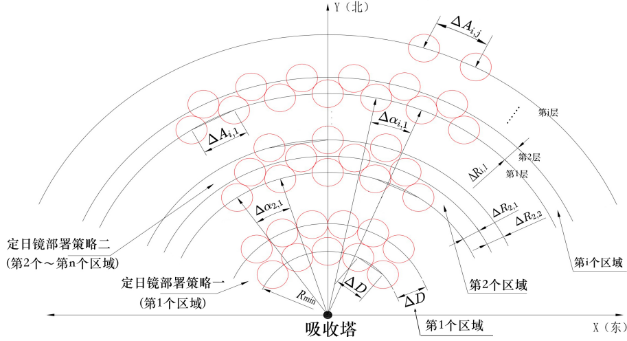
图 11: 区域划分示意图
