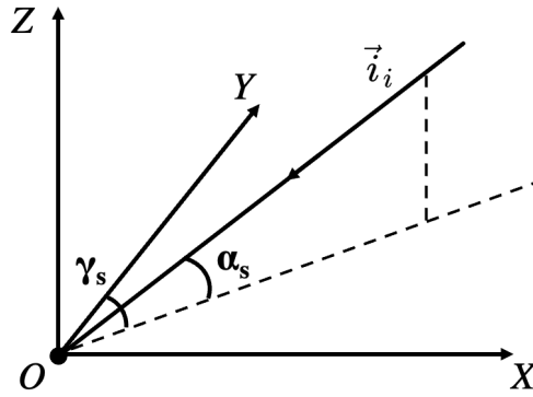
图 2: 镜场坐标系中入射光线示意图
