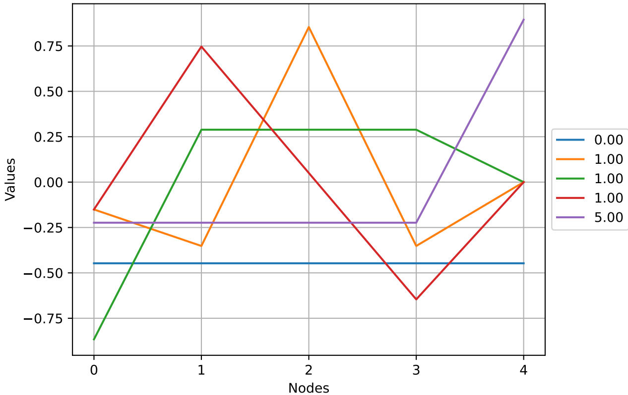
Eigenfunctions
