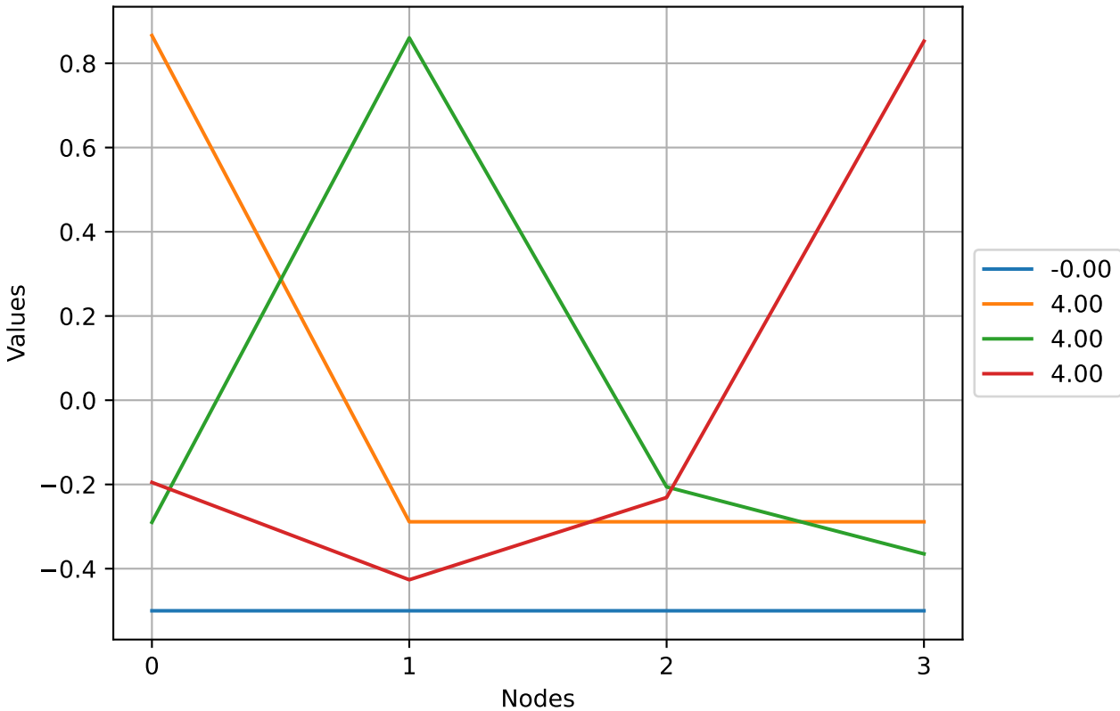
Eigenfunctions
