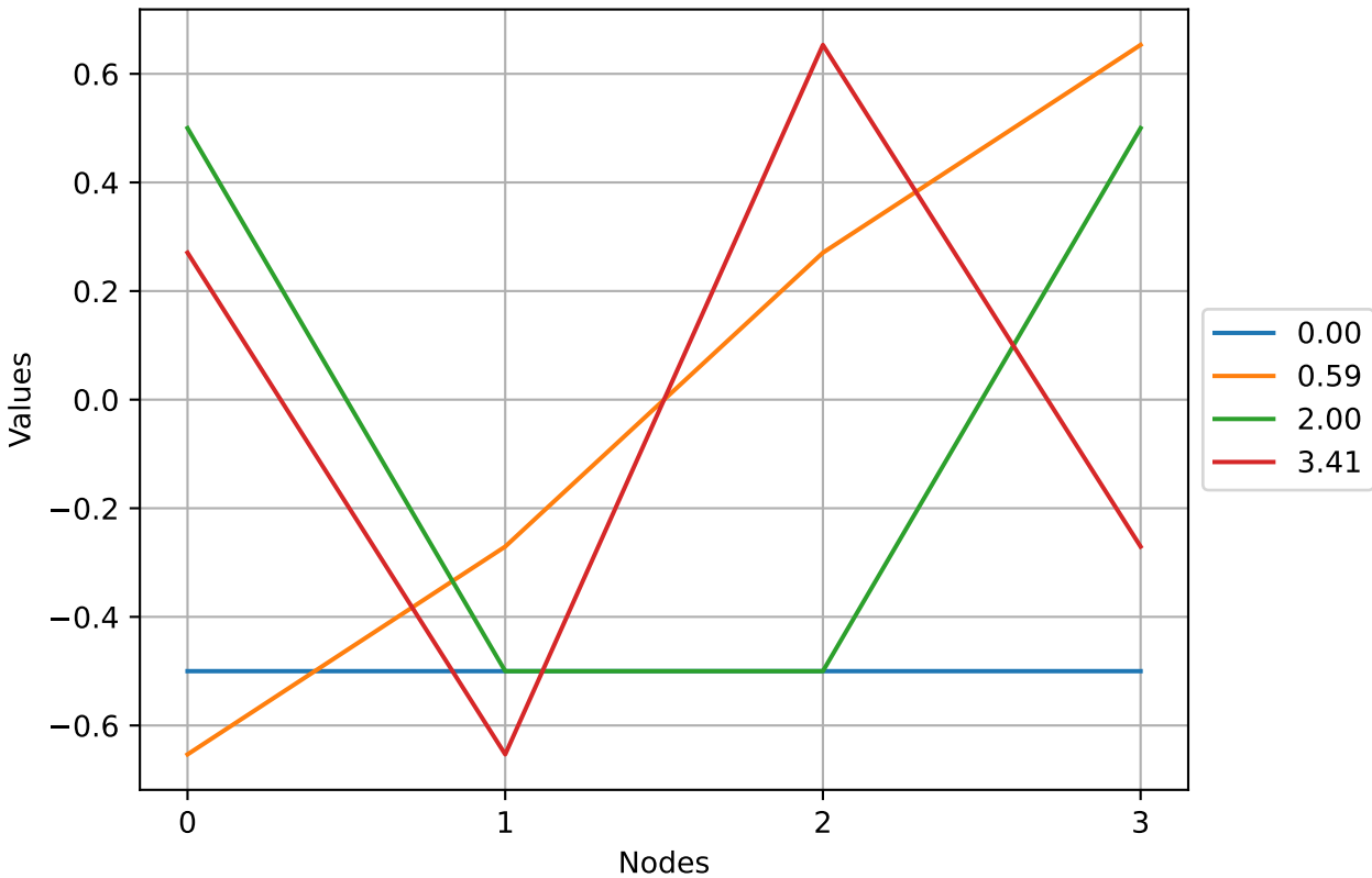
Eigenfunctions
