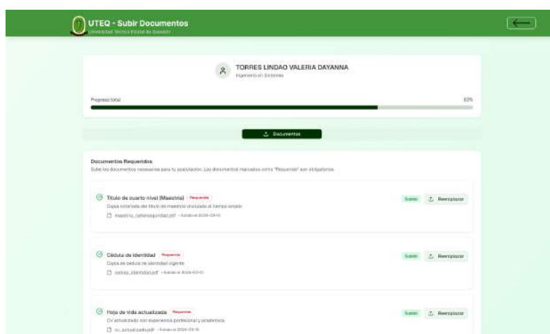
Figura 37: Interfaz de Subir documentos postulante
