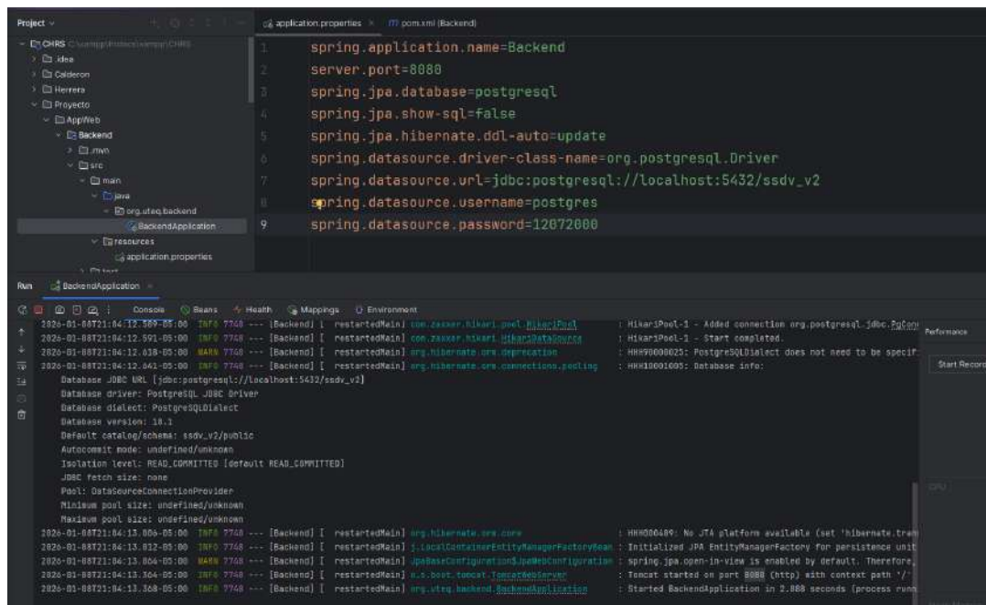
Figura 84: Configuración de Spring Boot y conexión exitosa a PostgreSQL
