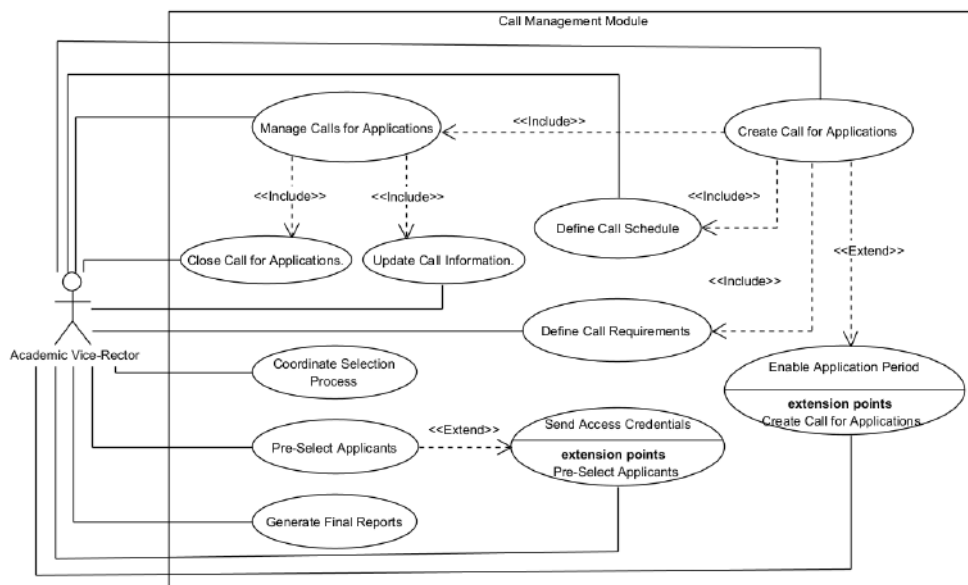
Figura 11: Módulo de Gestión de Convocatorias
