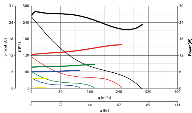
LINEO 100 ES
