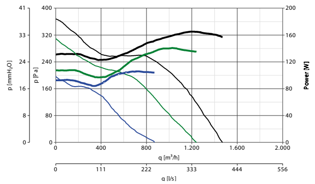
LINEO 250
