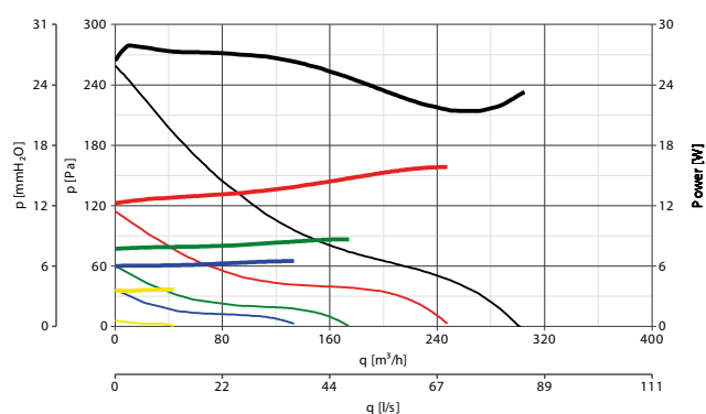
LINEO 150 ES
