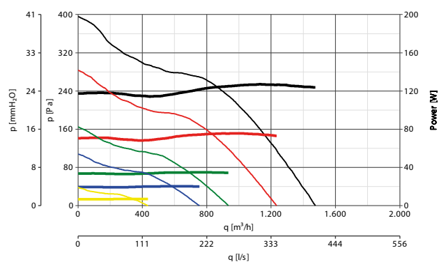
LINEO 250 ES
