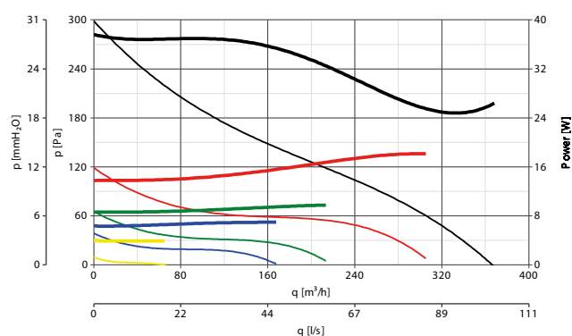
LINEO 125 ES
