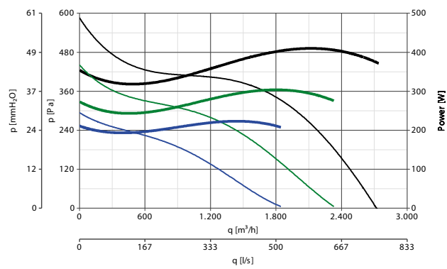
LINEO 315
