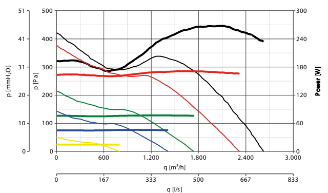
LINEO 315 ES
