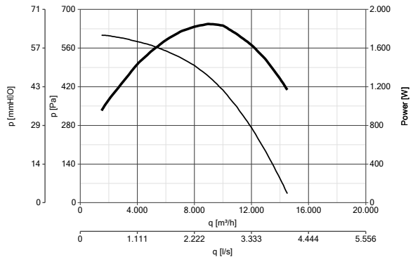
VORT QBK SAL-KC EVO 315 T2 1.5kW code 43164
