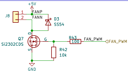
Fan connector
