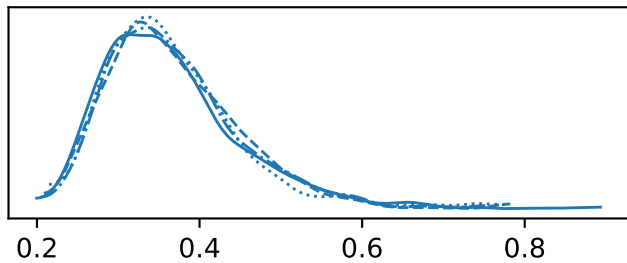
sigma_alpha
