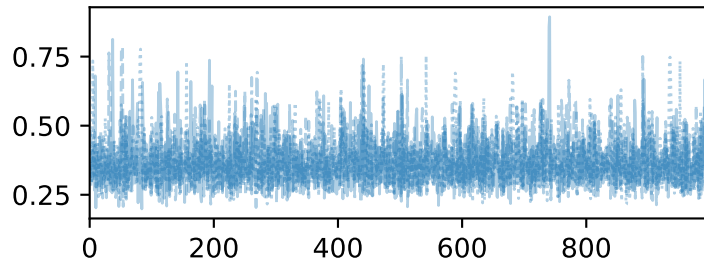
sigma_alpha
