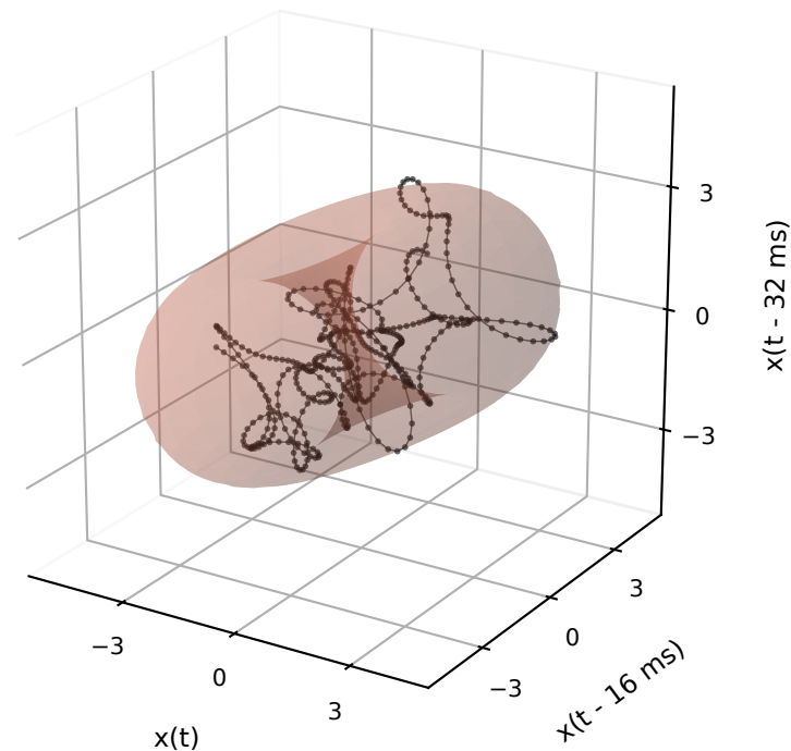
2-torus: donut volume
