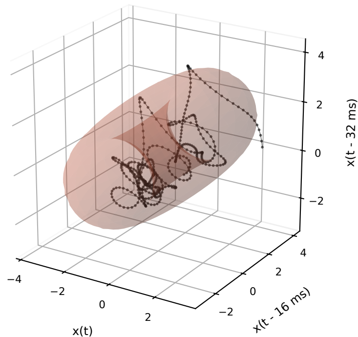
2-torus: donut volume
