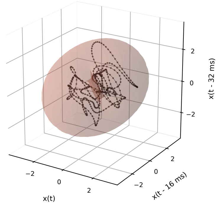
2-torus: donut volume
