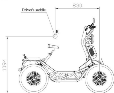
Variant SS: 1 Sitzplatz (Fahrersattel, R-Punkt)
