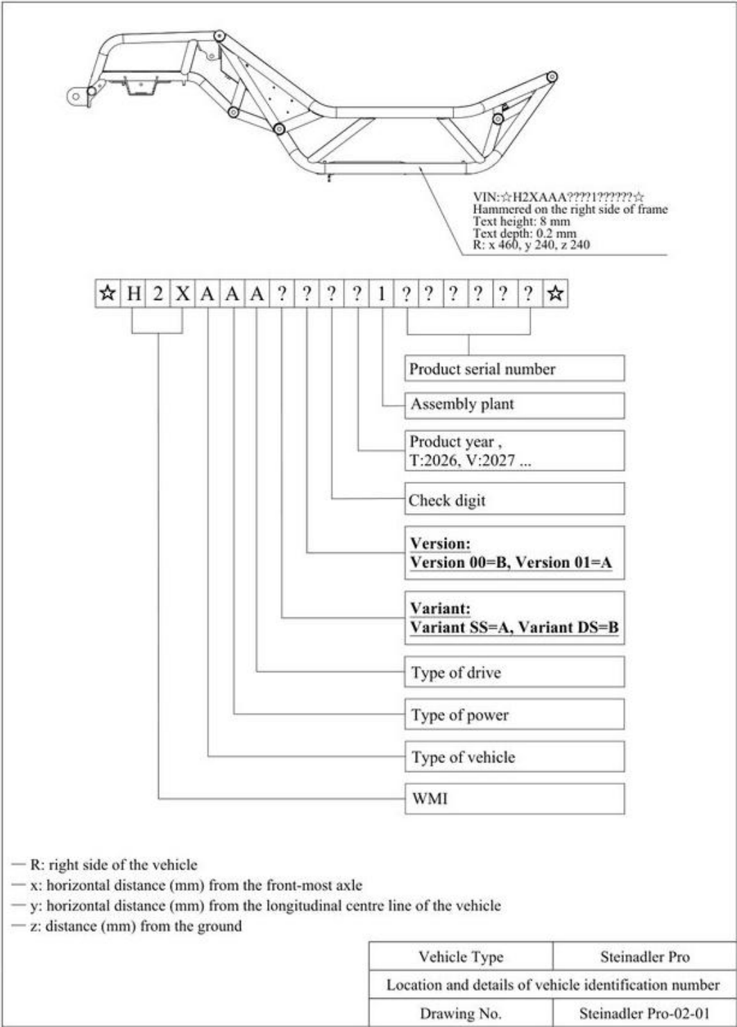
VIN-Position und Codierungsstruktur
