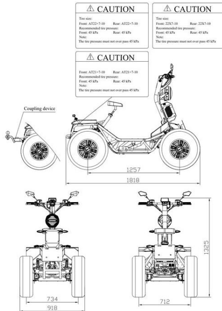
Variant SS – Fahrzeug-Maßzeichnung
