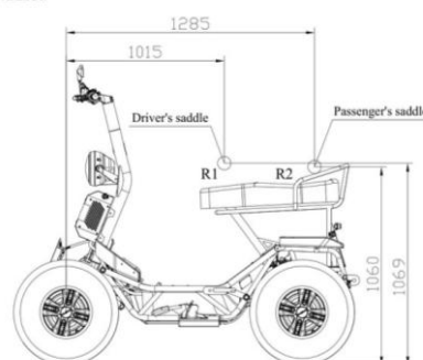
Variant DS: 2 Sitzplätze (Fahrer R1 + Beifahrer R2)
