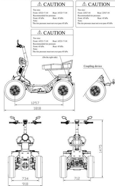
Variant DS – Fahrzeug-Maßzeichnung (Höhe 1475 mm)
