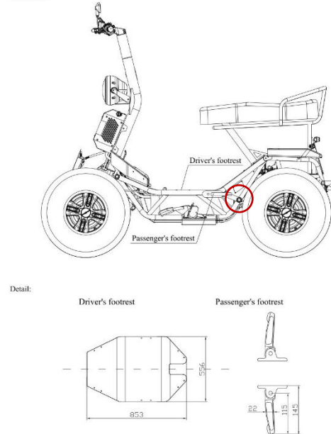
Variant DS: Fahrer- + Beifahrer-Fußraste (2×)
