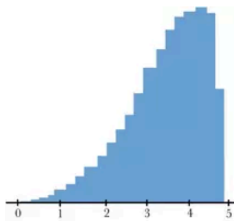
skew left
