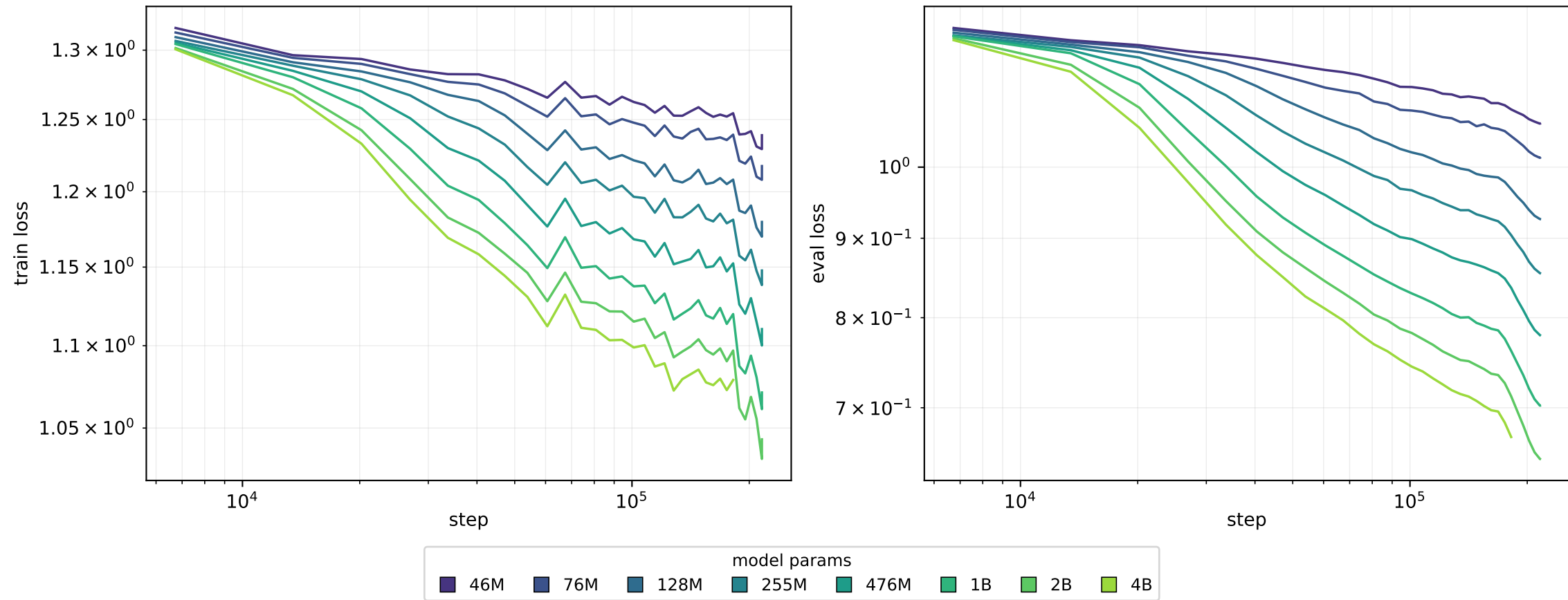
Parameter scaling — loss vs step
