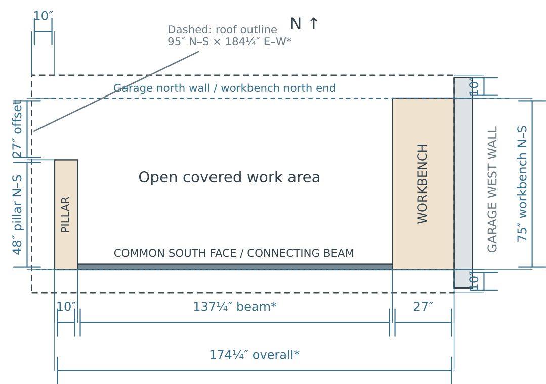
01 PLAN · north up
