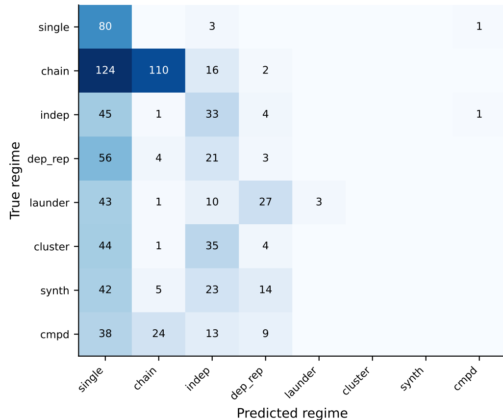
LLM (content-attentive)
