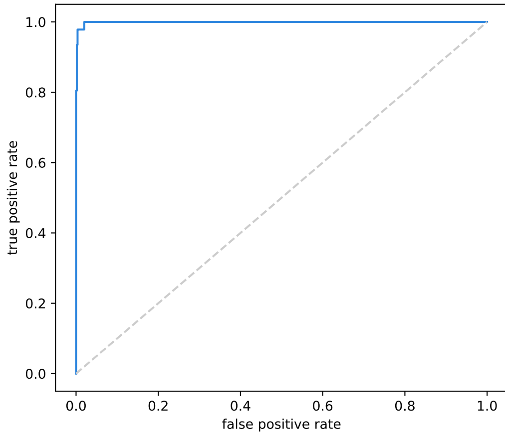
ROC (AUC = 0.999)
