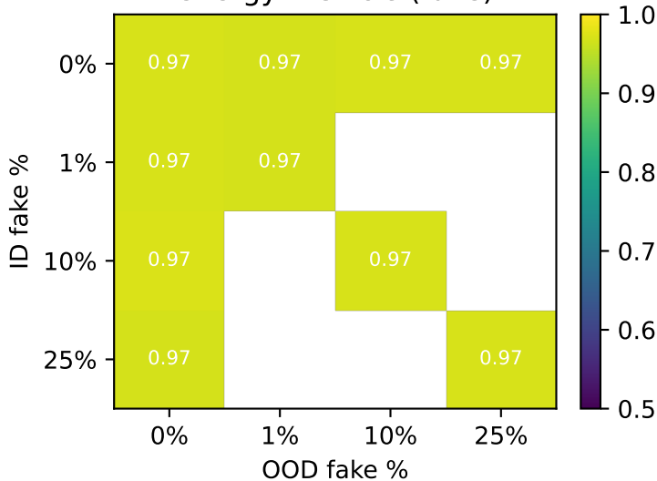
energy: AUROC (fake)
