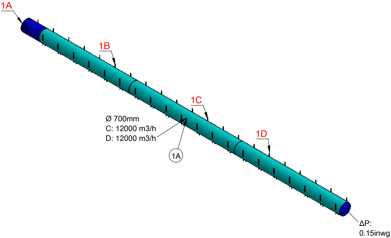
Vista isométrica
