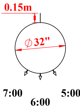
SECCIÓN A-A
