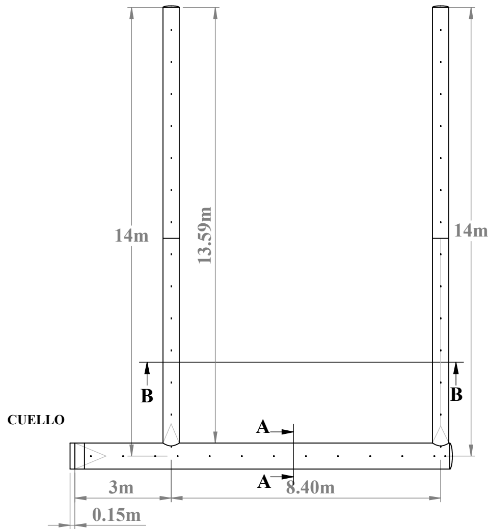
SOPORTES AJUSTABLES
