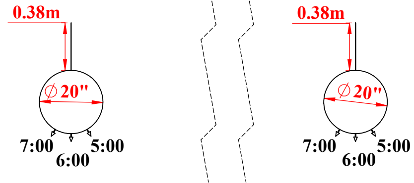
SECCIÓN B-B
