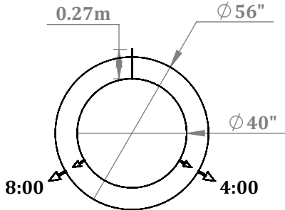
SECCIÓN B-B Ductos 2B-C,3C-D,4C-D,5C-D,6C-D,7A-B,8A-B,9A-B,10A-B,11A-B & 12A-B
