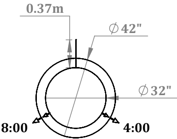
SECCIÓN A-A Ductos 1D,1E,1F & 1G
