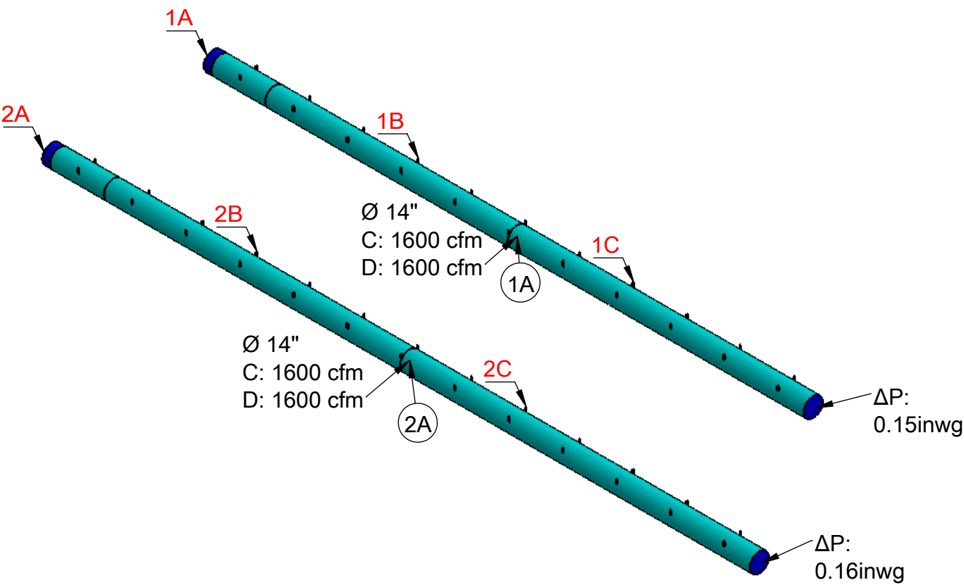
Vista isométrica
