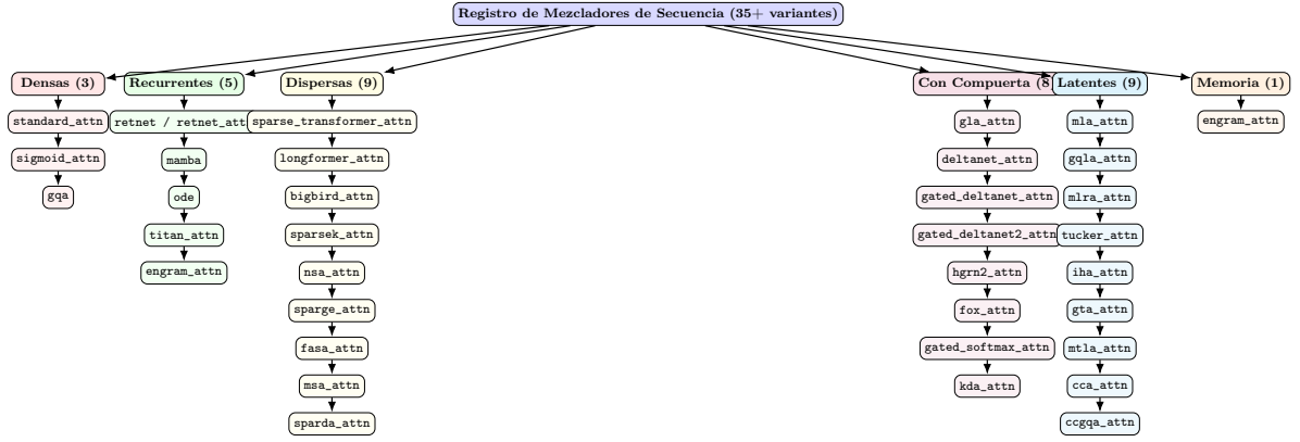
Figura 2: Taxonomía completa de treinta y cinco variantes de mezcladores de secuencia en seis categorías funcionales. Las líneas base densas proporcionan enrutamiento global completo a costo cuadrático. Las arquitecturas recurrentes permiten inferencia en tiempo constante mediante compresión de estado. Las variantes dispersas reducen la complejidad mediante patrones estructurados o selección de tokens. Los mecanismos con compuerta introducen control dependiente de datos sobre la retención y el olvido de memoria. Los métodos latentes comprimen representaciones clave-valor en cuellos de botella de rango bajo. La memoria condicional proporciona lectura/escritura en tiempo de prueba sobre un banco de memoria externo.
