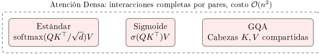
Figura 4: Tres líneas base de atención densa. La atención softmax estándar y la sigmoide calculan matrices QK^T completas. La Atención por Consultas Agrupadas (GQA) comparte cabezas clave-valor entre grupos de consultas, reduciendo el ancho de banda de memoria mientras preserva la expresividad completa de la atención.
