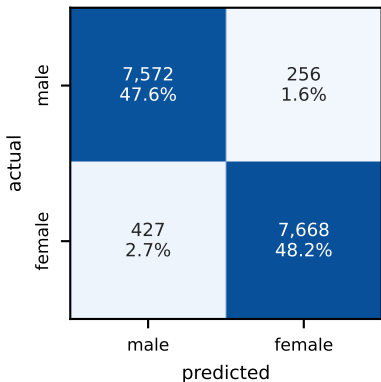
(b) CharBiGRU
