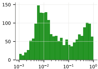
oracle MAP error (test)
