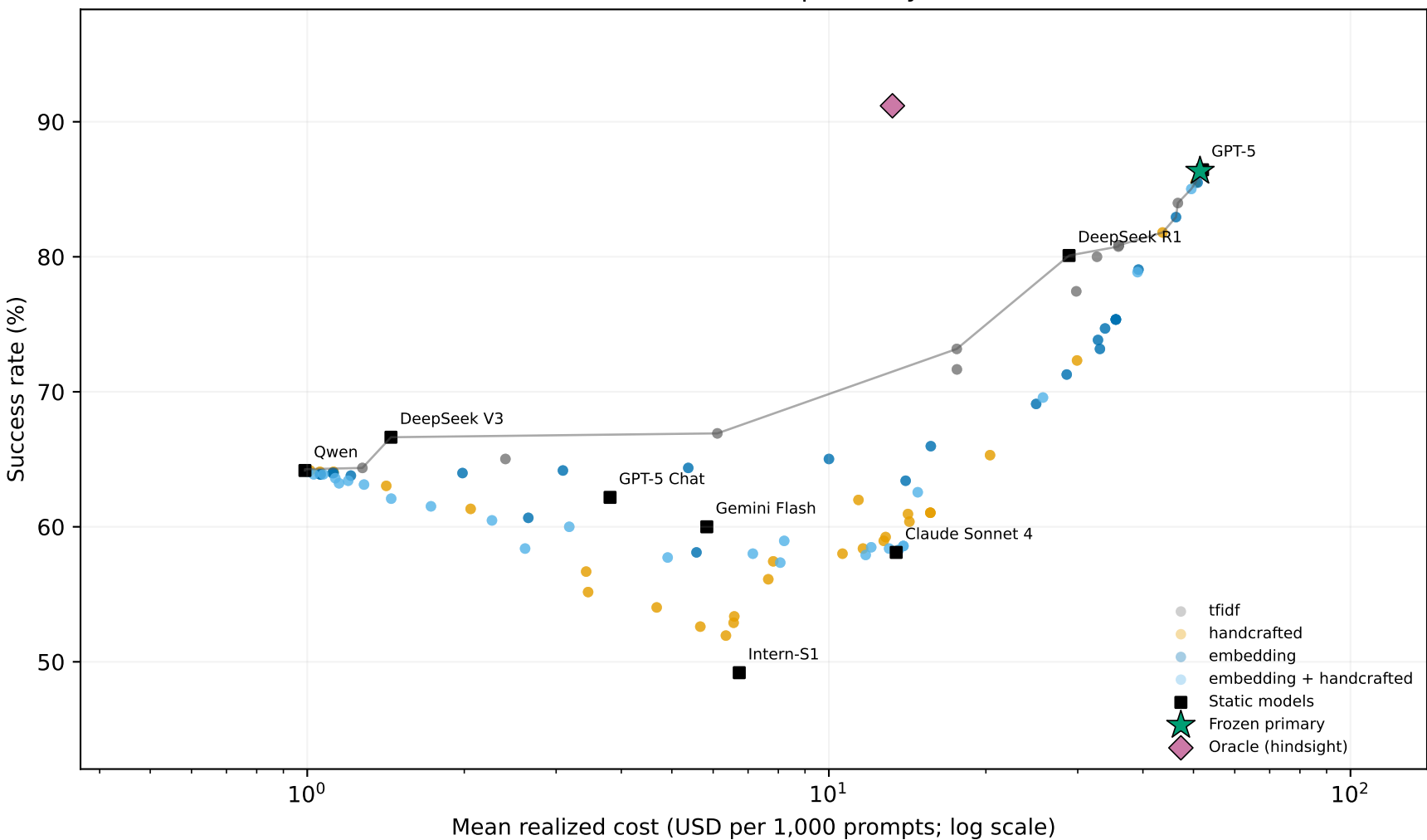
Router v2 — OOD exploratory test
