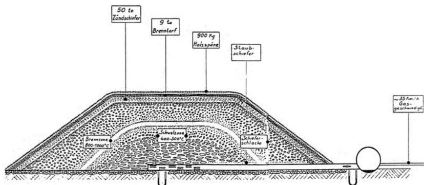
Querschnitt durch einen Schiefermeiler des Meilerverfahrens, welches das zentrale Verfahren des Unternehmens „Wüste“ war.
