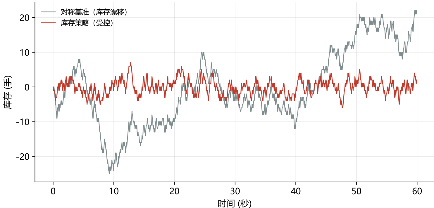
Track A (hftbacktest 真实撮合引擎)：A-S 报价下的库存路径
