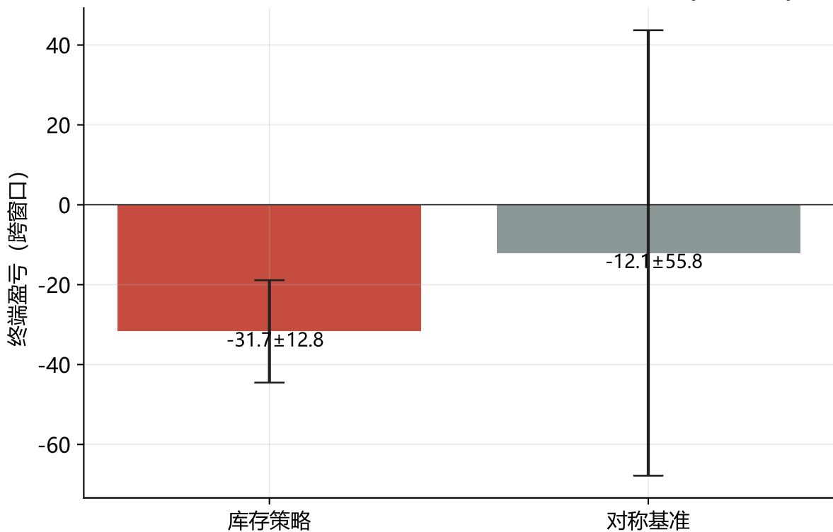
Track A 真实 Binance 数据：盈亏均值 \pm 跨窗口标准差 (4 个窗口)
