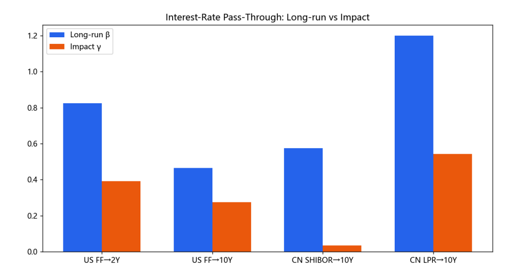
图 9：利率传导：长期 b 与即期 \gamma 对比。中国 SHIBOR→10Y 的即期传导极低。
