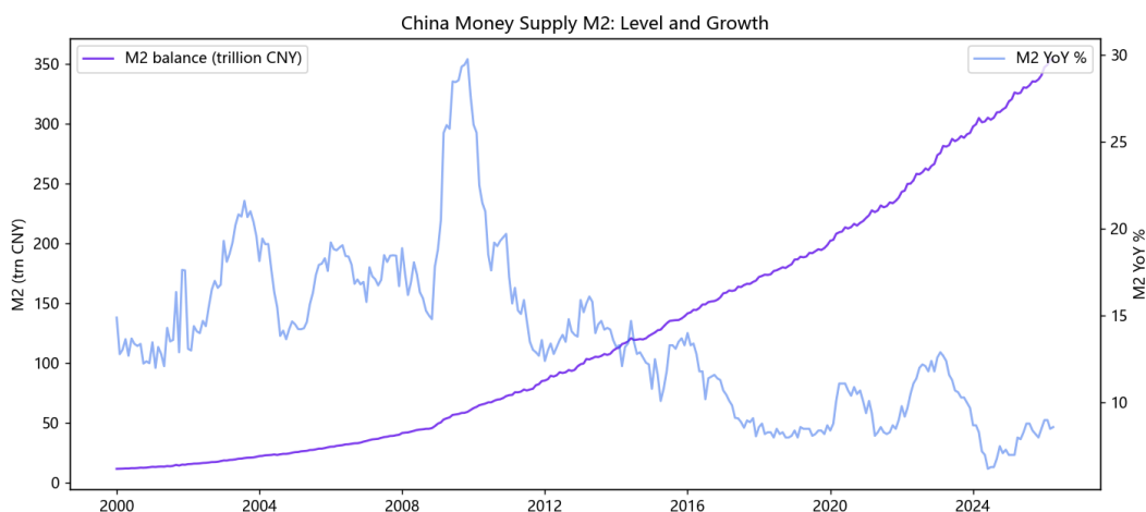
图 11：中国 M2 余额与增速：货币深化。
