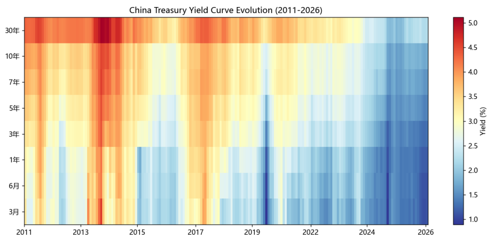
图 4：中国国债收益率曲线演变（2011–2026）。中枢更平稳，近年趋势性下移。
