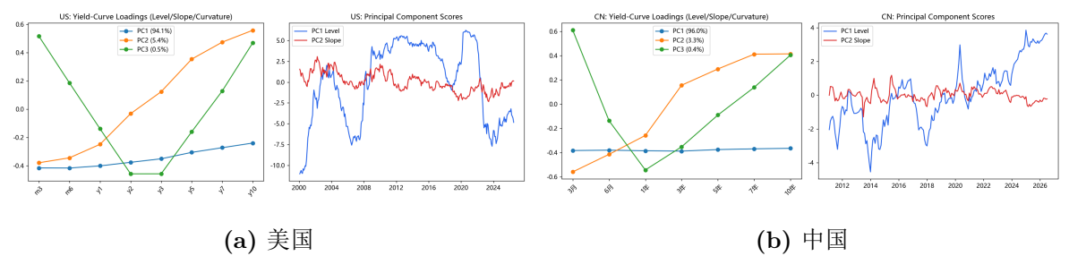
图 8：收益率曲线主成分（载荷与得分）：水平/斜率/曲率。
