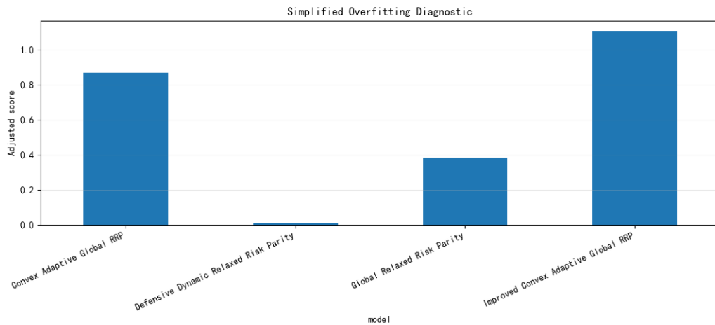
图 6-22 过拟合诊断
