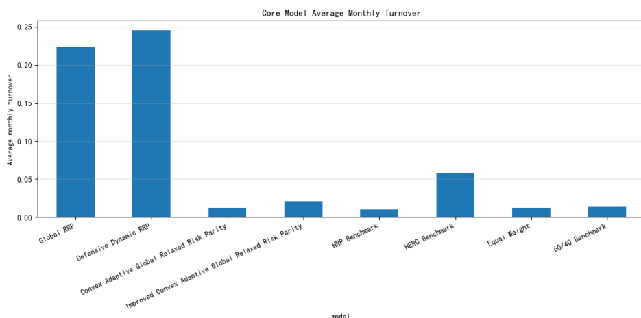
图 5-5 核心模型平均月度换手率比较
