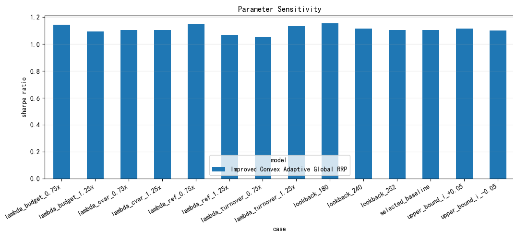
图 6-17 参数扰动敏感性检验
