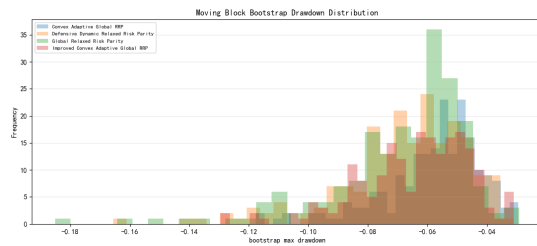
图 6-23 分块自助法最大回撤分布（200 个自助样本）
