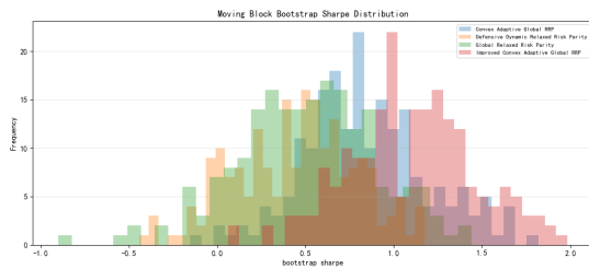
图 6-22 分块自助法夏普比率分布（200 个自助样本）
