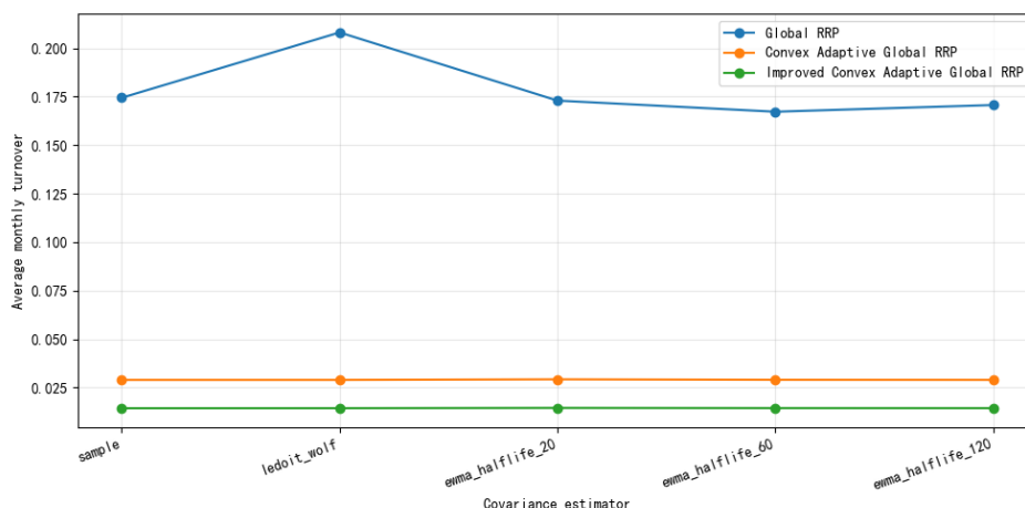
图 6-20 不同协方差估计下的换手表现
