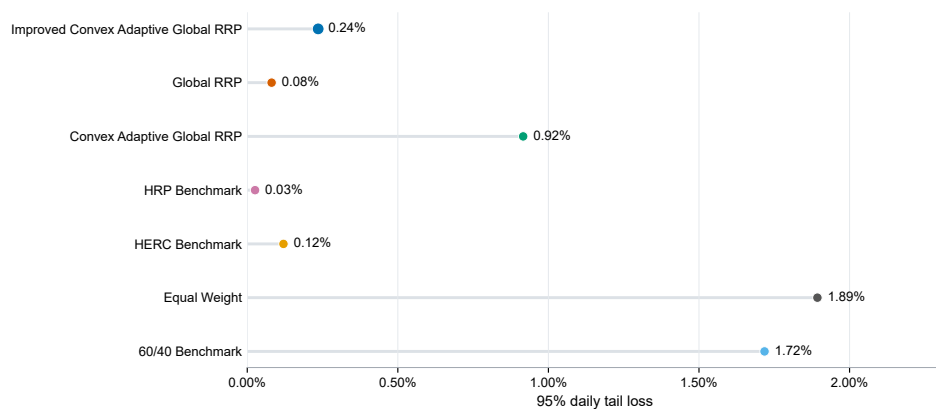
图 5-6 核心模型历史尾部损失
