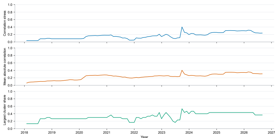
图 4-1 资产池跨类别相关结构
