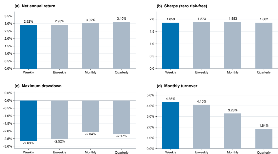
图 6-7 主模型参数下的调仓频率比较
