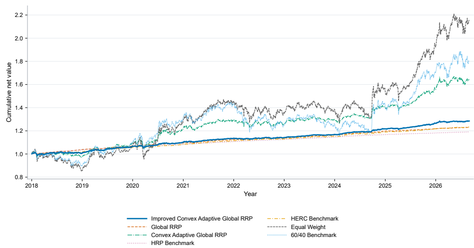
图 5-2 主模型与对照累计净值
