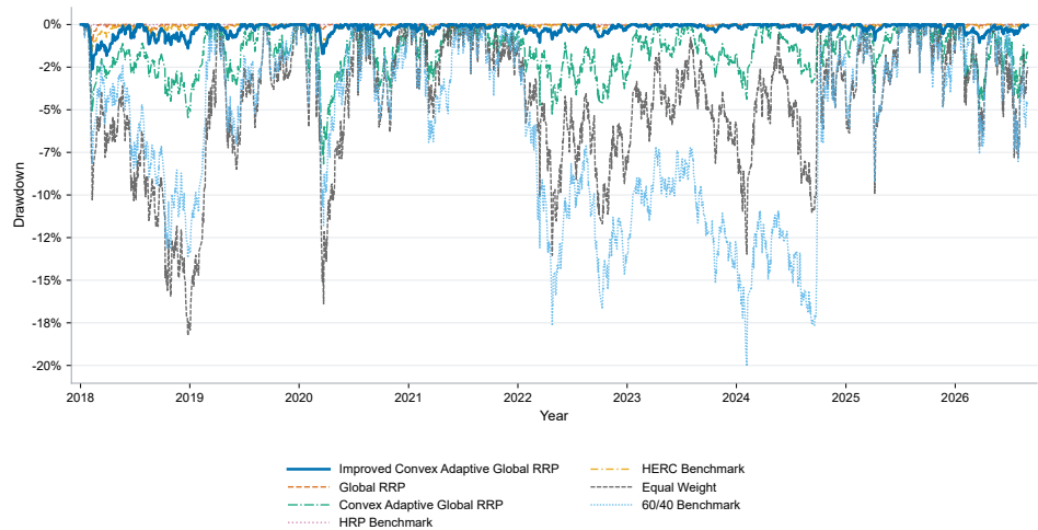
图 5-3 主模型与对照回撤
