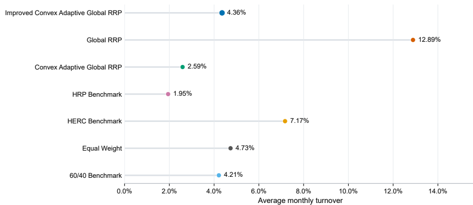
图 5-4 按自然月汇总的平均换手
