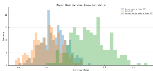
图 6-23 分块自助法夏普比率分布（200 个自助样本）
