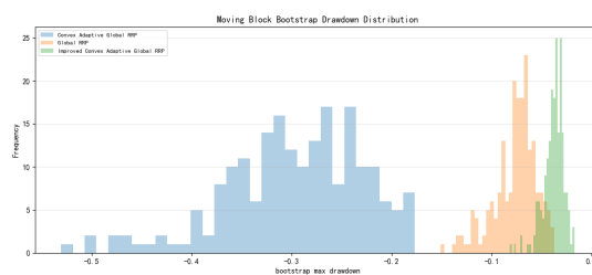
图 6-24 分块自助法最大回撤分布（200 个自助样本）
