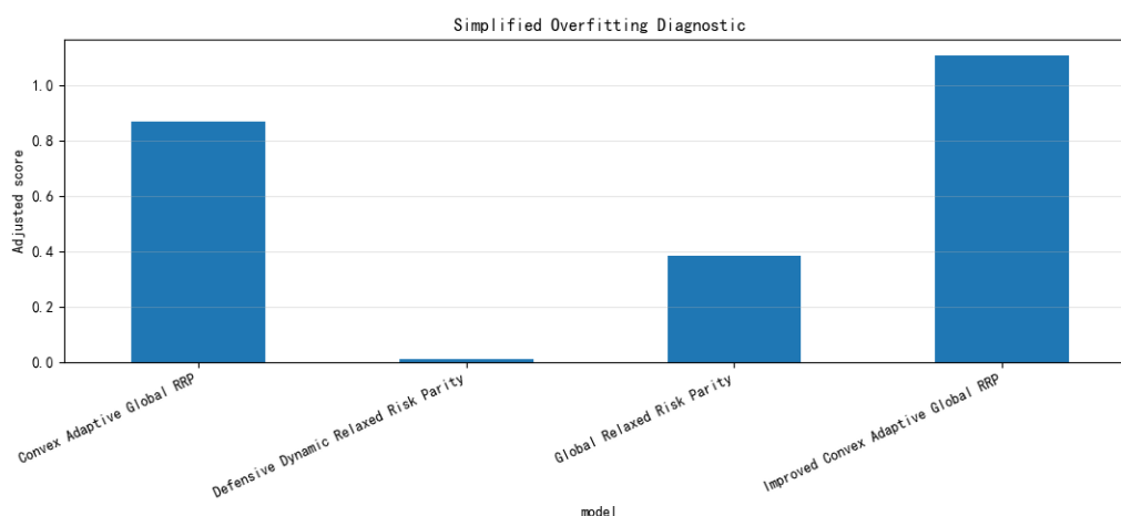
图 6-22 过拟合诊断
