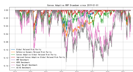
图 5-4 核心模型回撤路径比较
