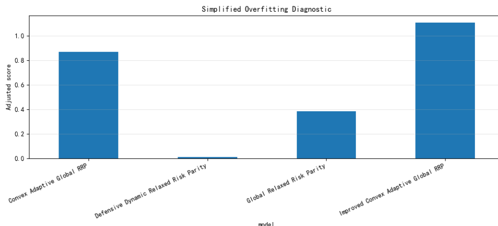
图 6-21 过拟合诊断
