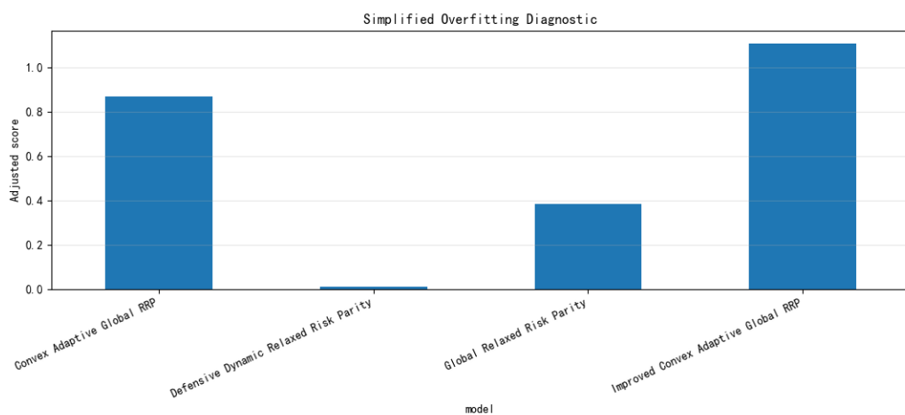
图 6-20 过拟合诊断
