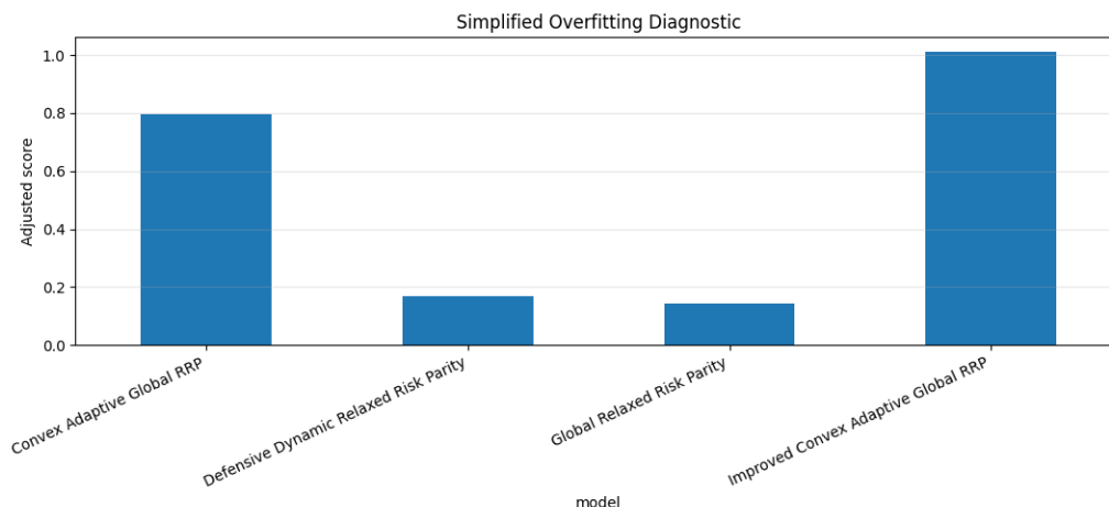
图 6-22 过拟合诊断
