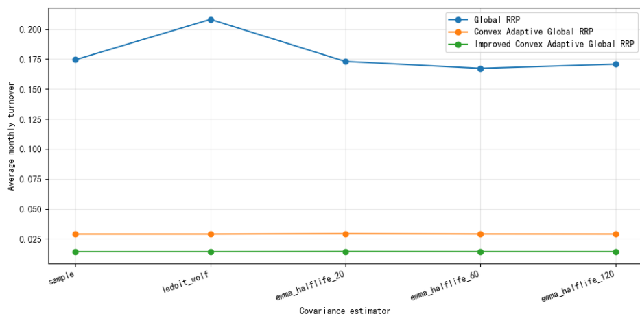
图 6-18 不同协方差估计下的换手表现
