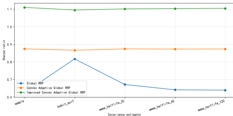
图 6-16 不同协方差估计下的夏普比率
