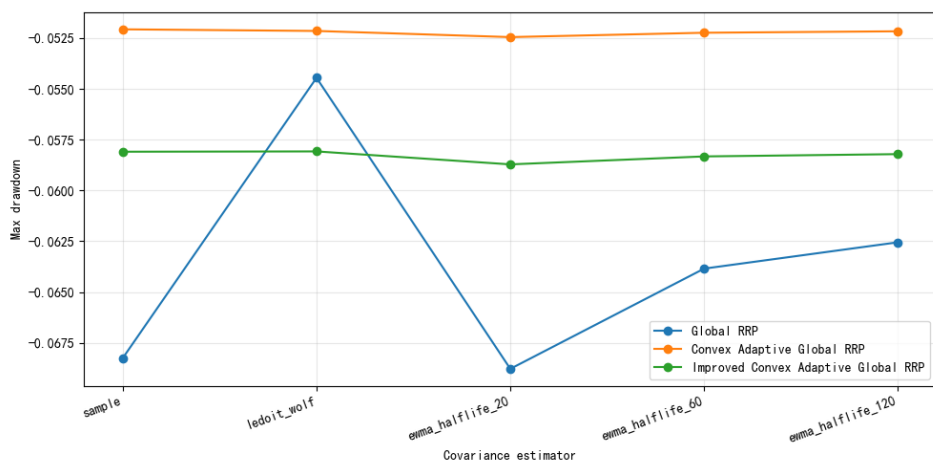
图 6-17 不同协方差估计下的回撤表现
