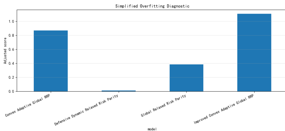
图 6-19 过拟合诊断
