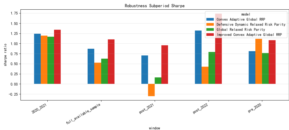
图 6-11 子区间夏普比率稳健性
