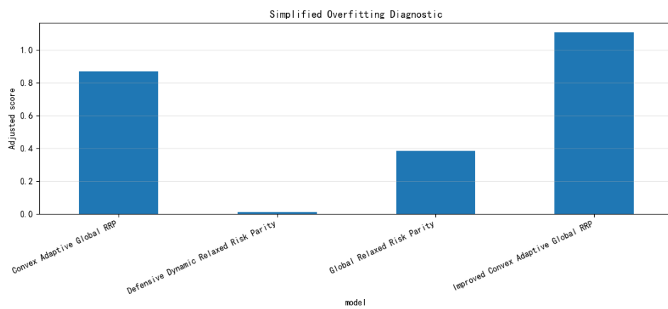
图 6-19 过拟合诊断
