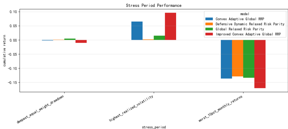
图 6-13 压力期表现检验
