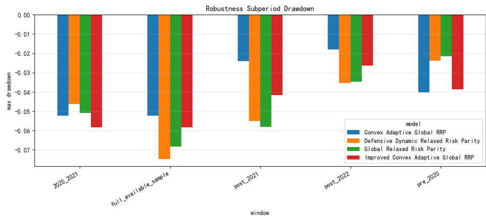
图 6-12 子区间最大回撤稳健性
