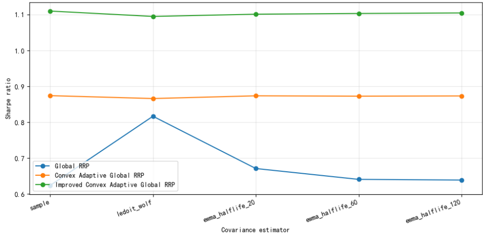
图 6-16 不同协方差估计下的夏普比率
