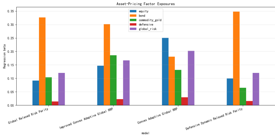
图 5-7 核心模型因子暴露汇总（全样本回归）
