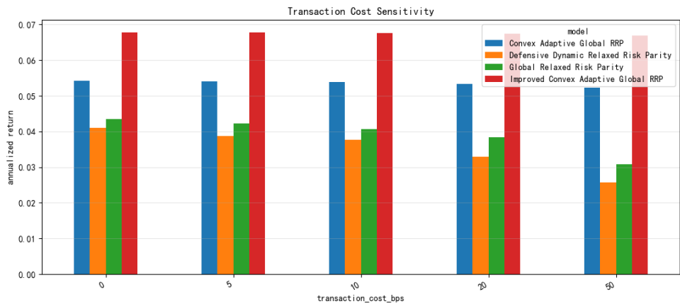
图 6-14 交易成本敏感性检验
