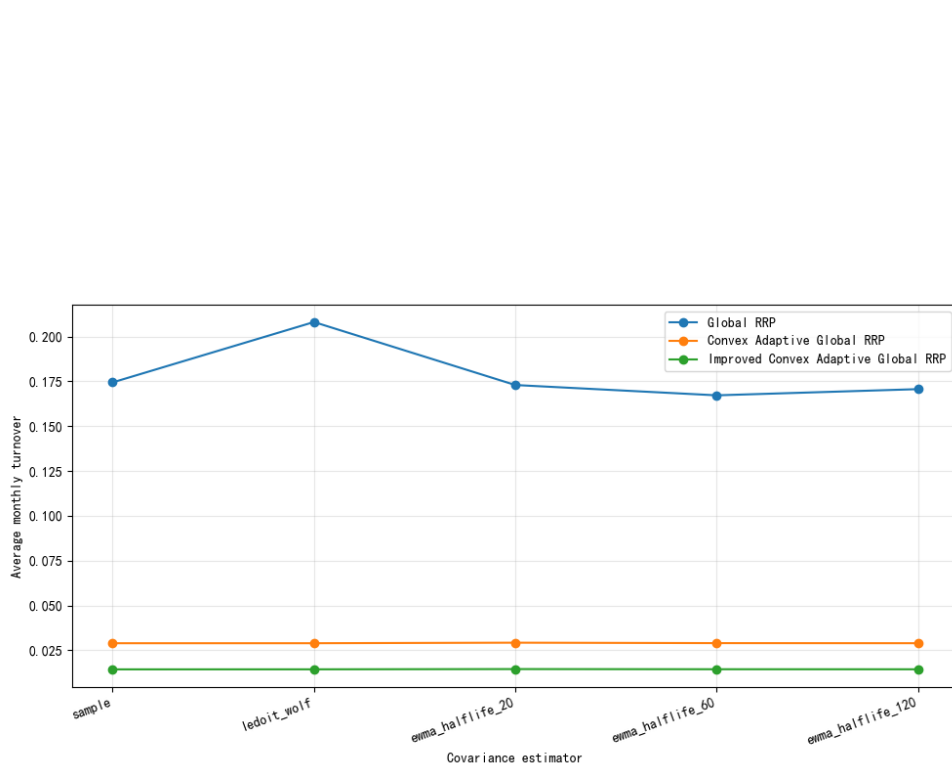
图 6-18 不同协方差估计下的换手表现
