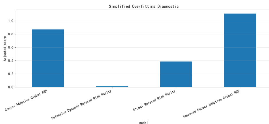
图 6-17 过拟合诊断
