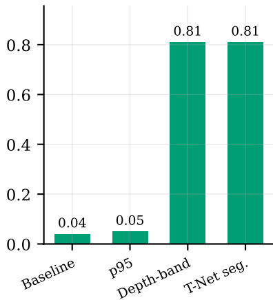
AMOTA ↑
