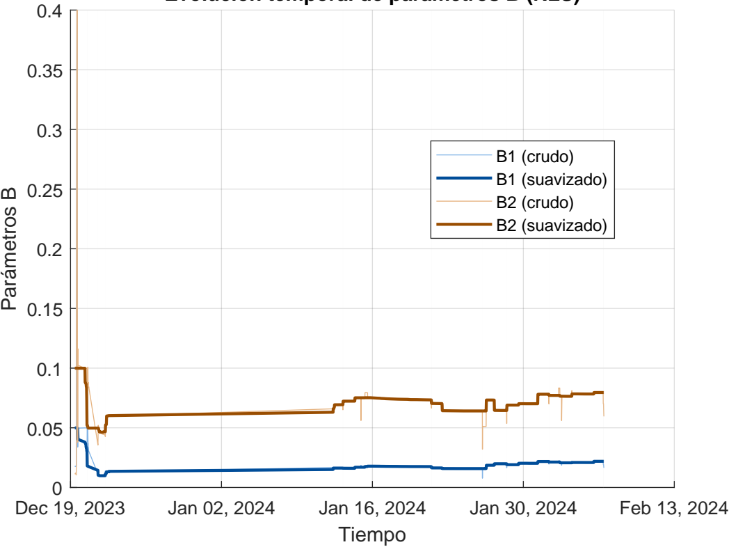
Evolución temporal de parámetros B (RLS)
